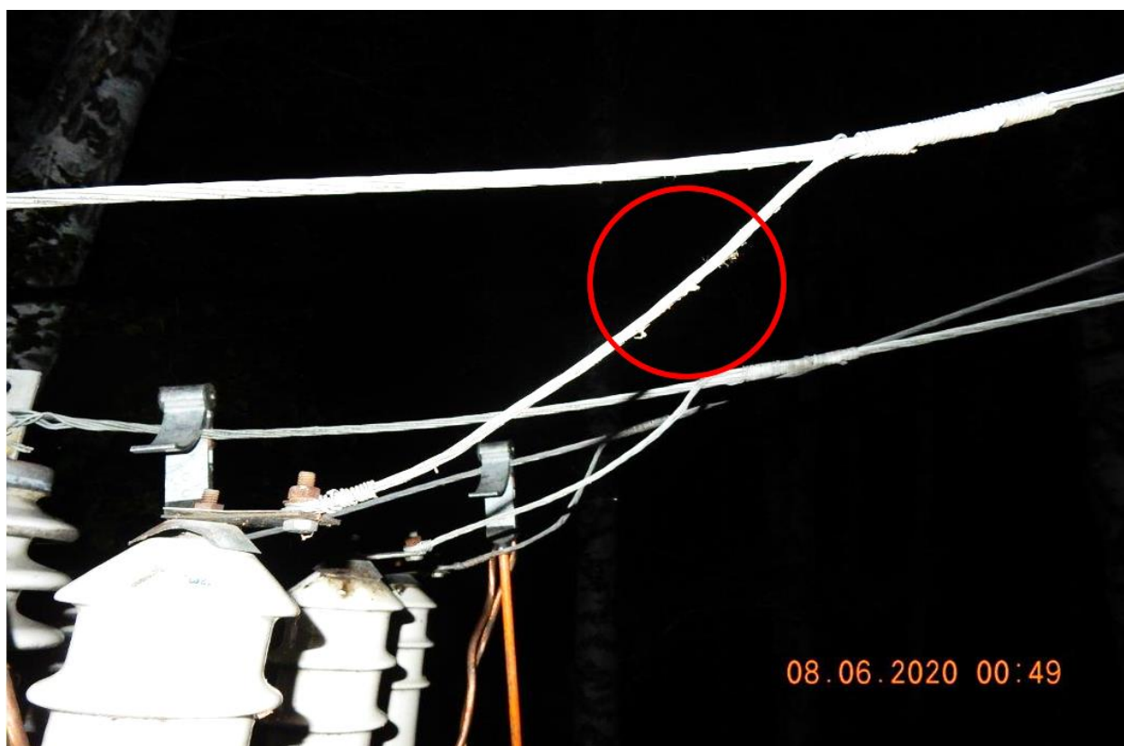
Фотография № 5. Следы воздействия электрической дуги на проводе.
