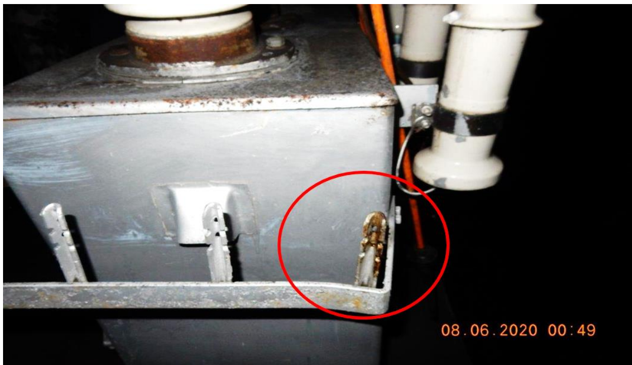
Фотография № 4. Следы воздействия электрической дуги.
